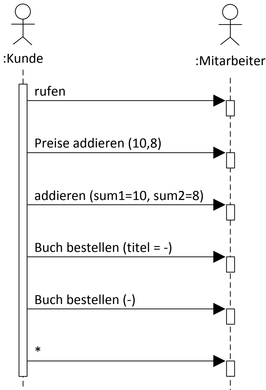
Abbildung 61: Argumentübertragung bei Nachrichten
