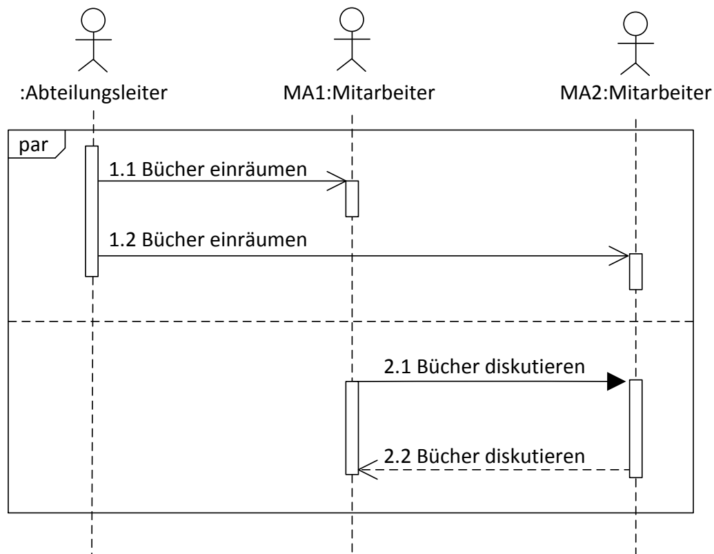
Abbildung 66: Darstellung von parallelen Nachrichtenflüssen
