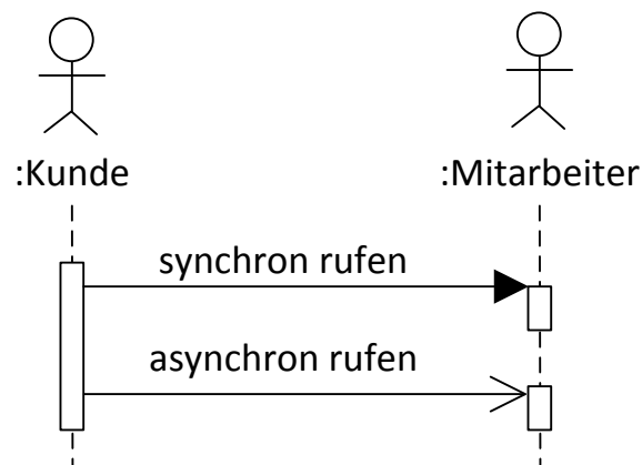
Abbildung 56: Darstellung von synchroner und asynchroner Kommunikation zwischen einem Kunden und einem Mitarbeiter
