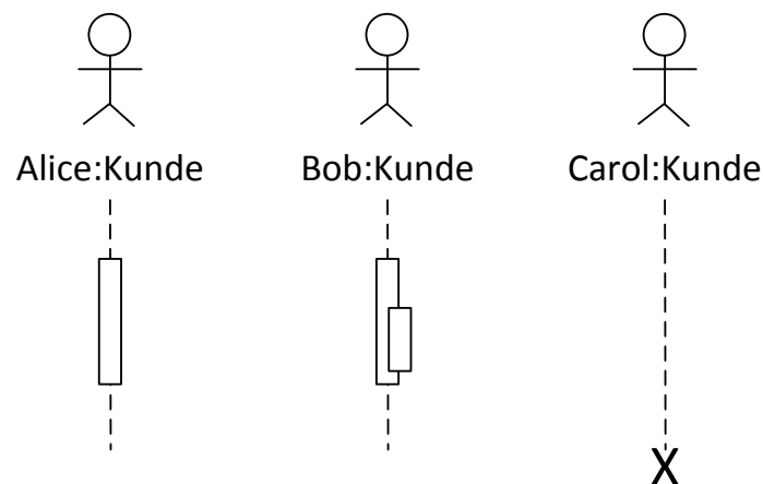
Abbildung 54: Drei Varianten der Lebenslinien mit Ausführungsbalken und Beendigung
