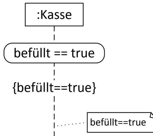
Abbildung 55: Die Zustandsinvariante von Lebenslinien
