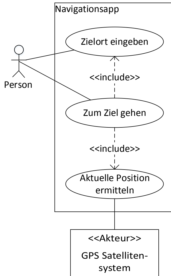
Abbildung 21: Anwendungsfalldiagramm des Navigationsbeispiels
