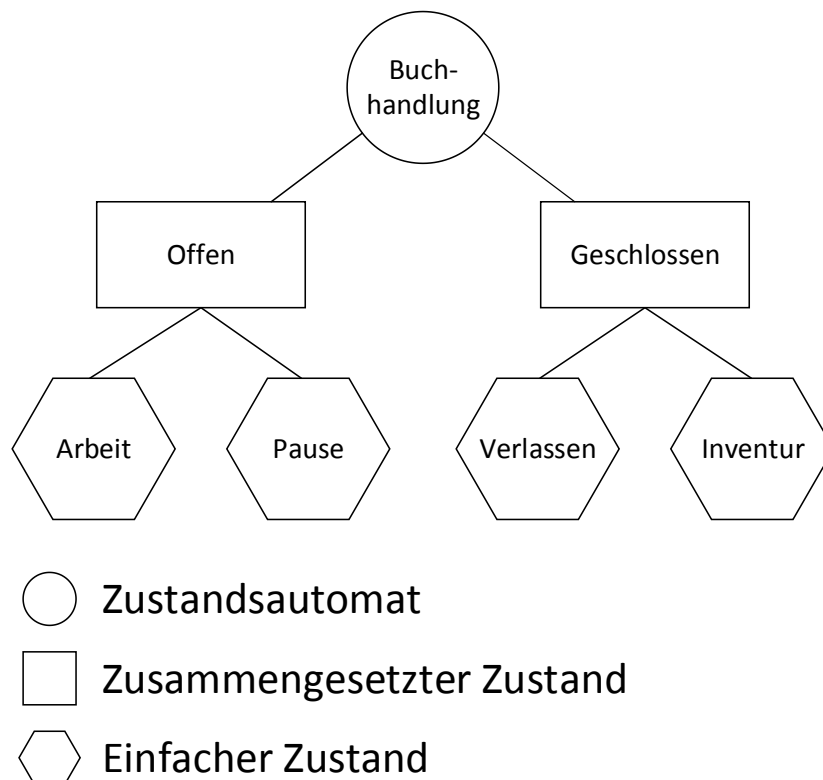
Abbildung 43: Darstellung sieben hierarchischer Zustände als Baum
