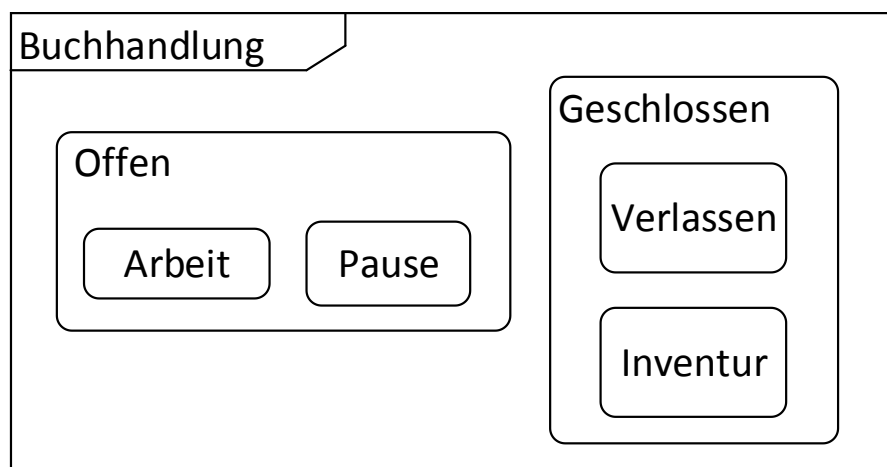
Abbildung 44: Beispielhafte Darstellung der hierarchischen Zustände des Baumes als Zustandsdiagramm
