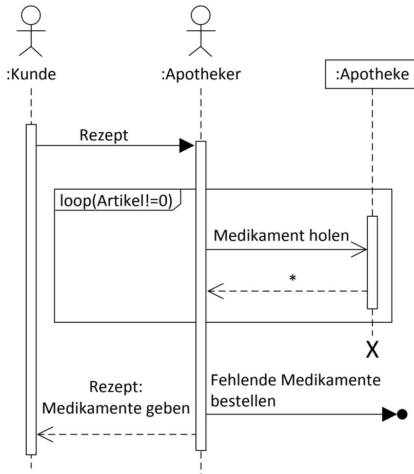
Abbildung A 5: Lösungsvorschlag für das Sequenzdiagramm
