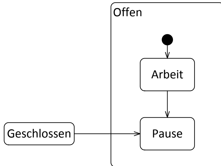
Abbildung 47: Explizites Betreten eines Unterzustands in einem zusammengesetzten Zustand
