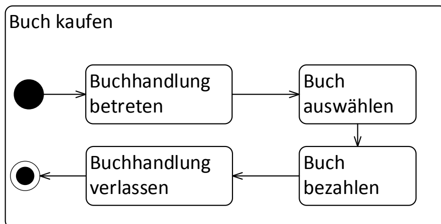
Abbildung 27: Beispiel der Aktivität „Buch kaufen“ bestehend aus mehreren Aktionen
