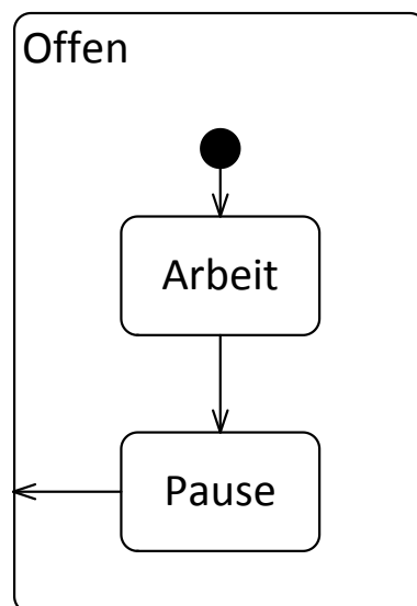
Abbildung 46: Zweite Variante des Standard-Eintritts
