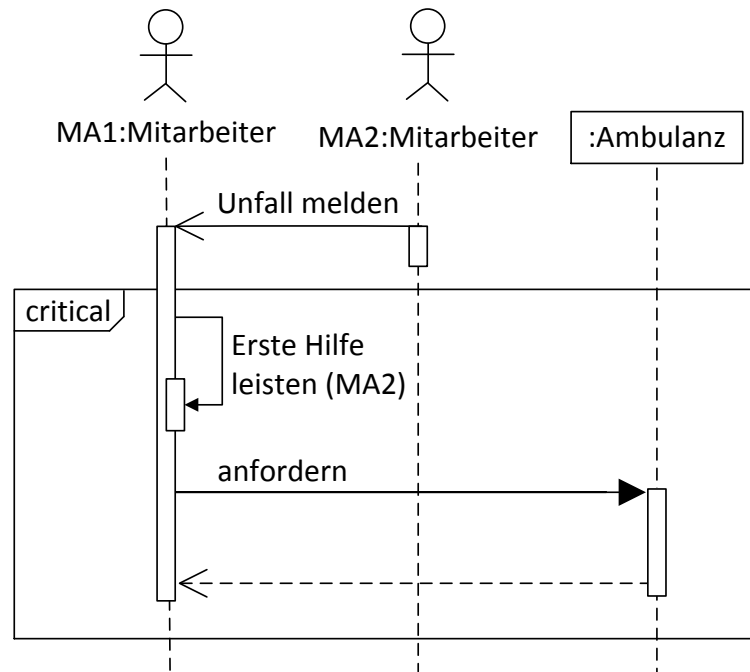
Abbildung 67: Darstellung eines nicht unterbrechbaren Bereichs "critical"
