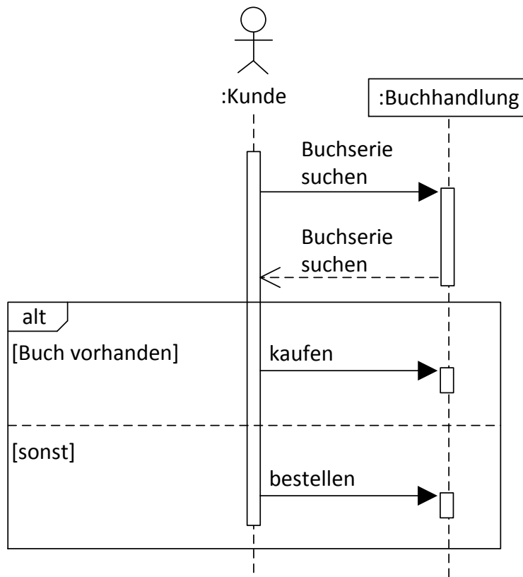
Abbildung 64: Darstellung von alternativen Nachrichtenflüssen
