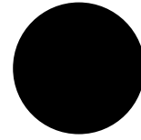
Abbildung 37: Startzustand
