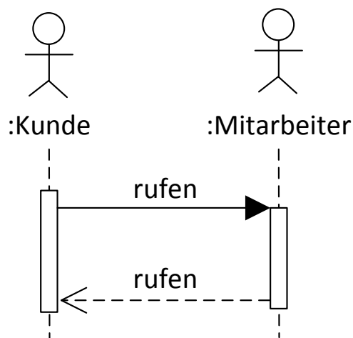
Abbildung 58: Die Antwortnachricht
