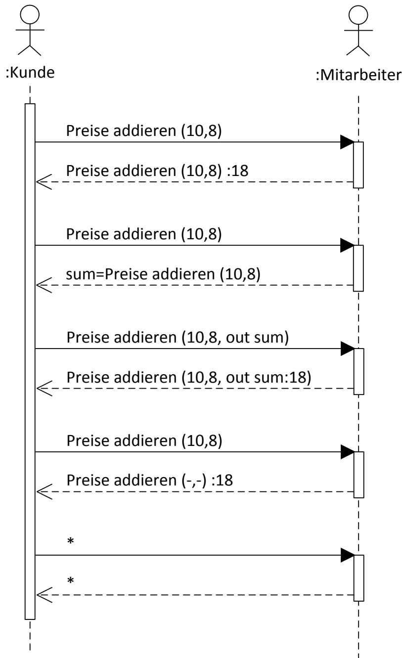
Abbildung 62: Rückgabewerte von Nachrichten mit Argumenten
