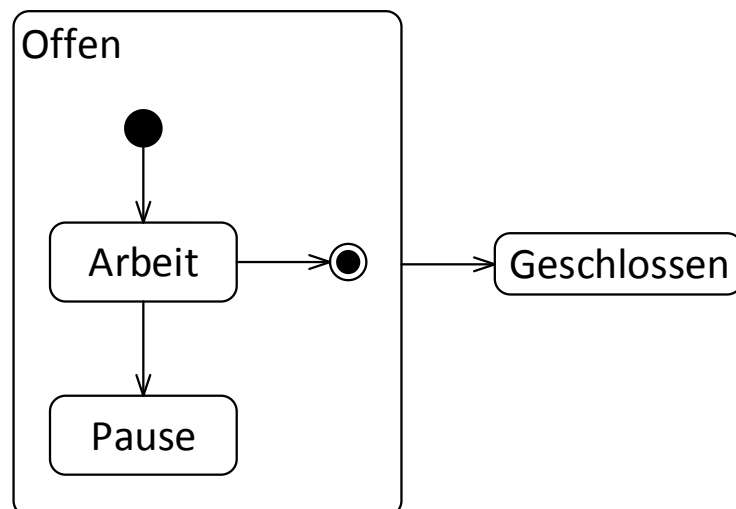
Abbildung 48: Verlassen eines zusammengesetzten Zustands mithilfe eines modellierten Endzustand
