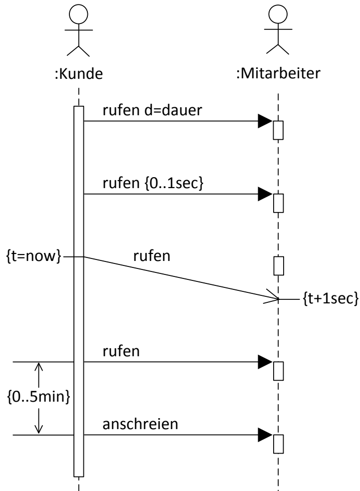
Abbildung 60: Modellierung von Zeitbedingungen von Nachrichten
