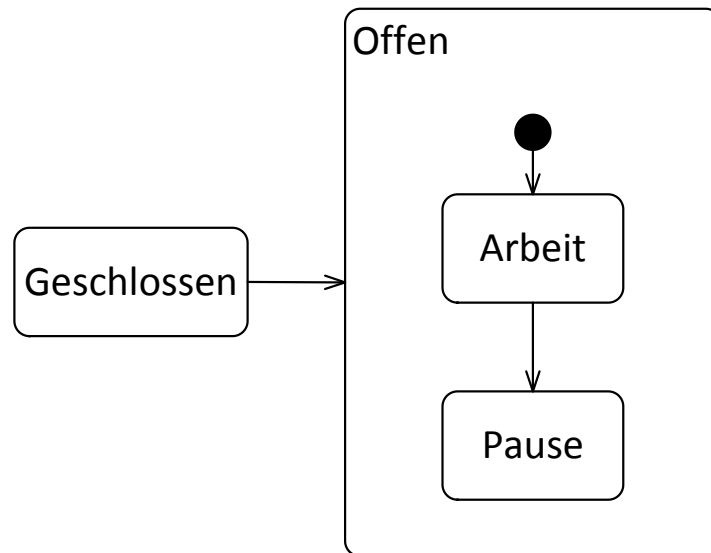
Abbildung 45: Standardeintritt in einen zusammengesetzten Zustand
