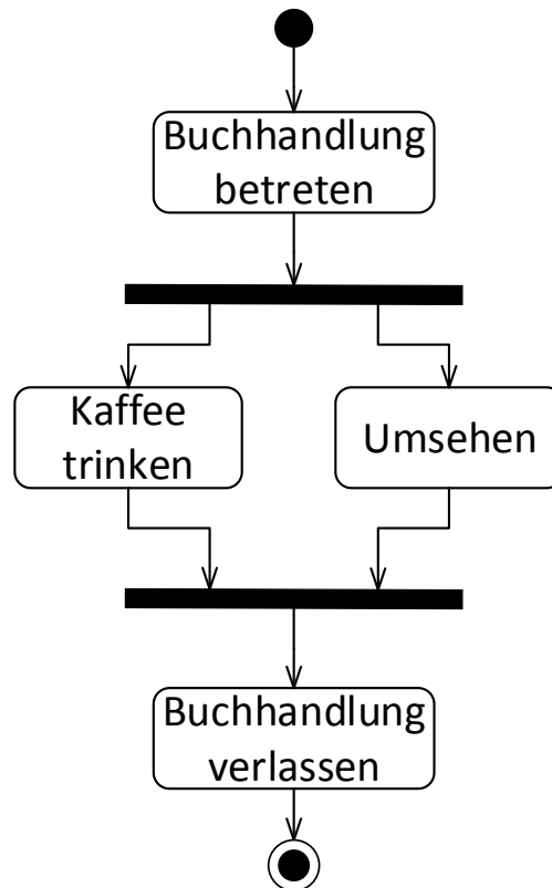
Abbildung 33: Beispiel paralleler Kontrollflüsse
