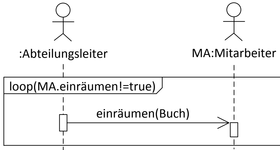
Abbildung 68: Mehrfache Durchführung von Interaktionen: die Schleife
