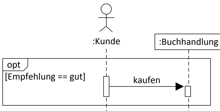
Abbildung 65: Optionale Nachrichtenflüsse anhand von Bedingungen
