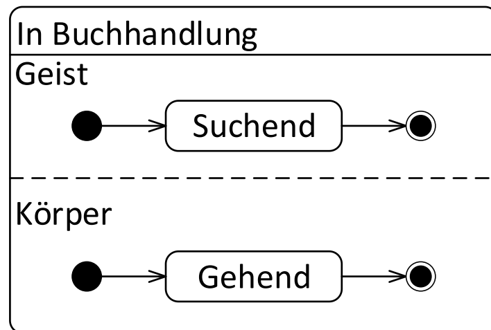
Abbildung 51: Orthogonaler Zustand „In Buchhandlung“ mit zwei Regionen „Geist“ und „Körper“
