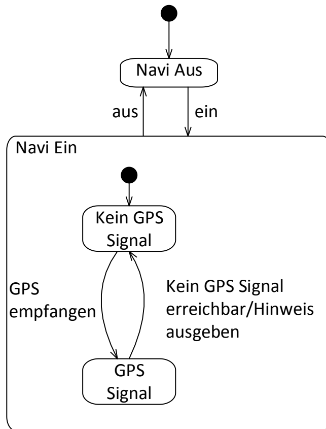
Abbildung 52: Zustandsdiagramm des Navigationsbeispiels
