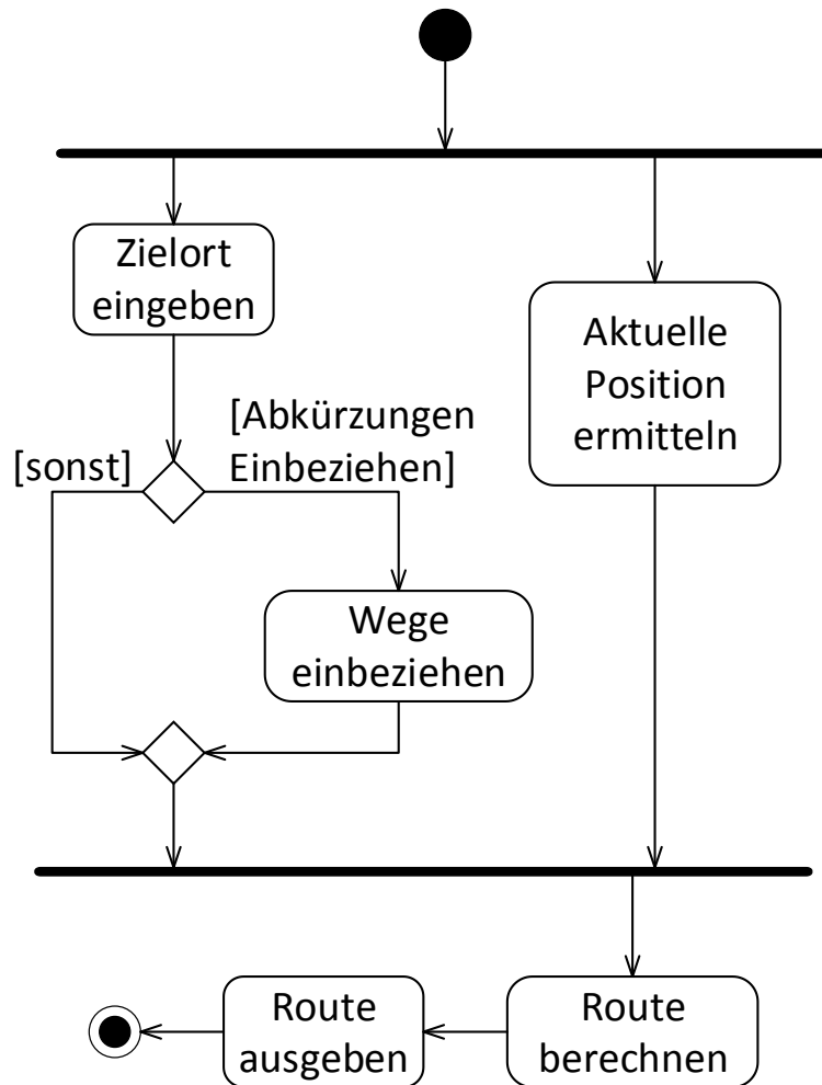
Abbildung 35: Aktivitätsdiagramm des Navigationsbeispiels
