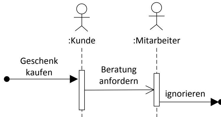
Abbildung 59: Gefundene und verlorene Nachrichten
