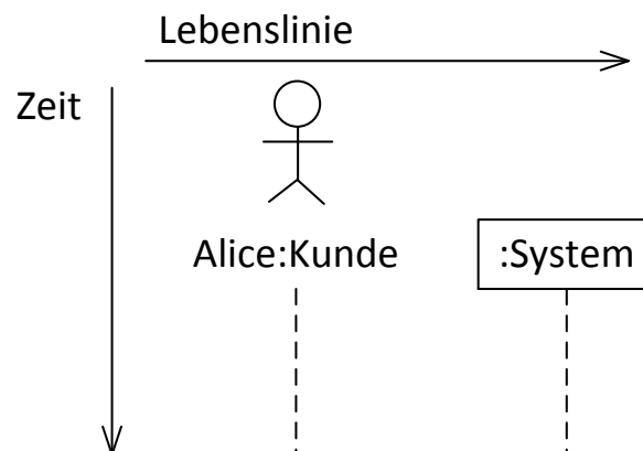
Abbildung 53: Die Zeit- und Interaktionsachse mit zwei Teilnehmern
