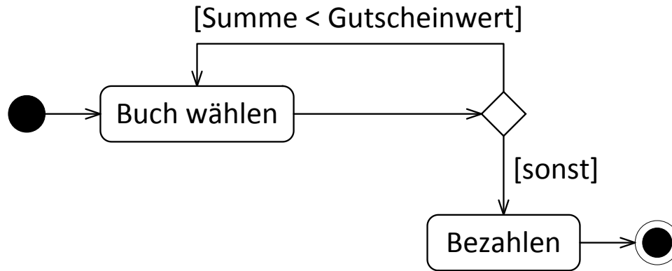
Abbildung 31: Darstellung einer Schleife durch bedingte Verzweigungen
