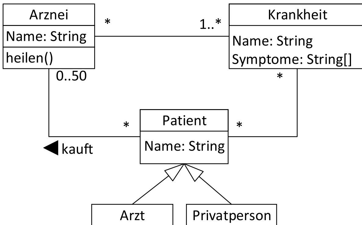
Abbildung A 1: Lösungsvorschlag für das Klassendiagramm
