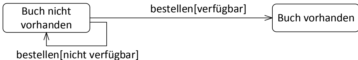
Abbildung 41: Transition zwischen zwei Zuständen mit Events und Guards
