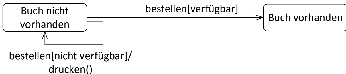
Abbildung 42: Transition zwischen zwei Zuständen mit Event, Guard und Aktion
