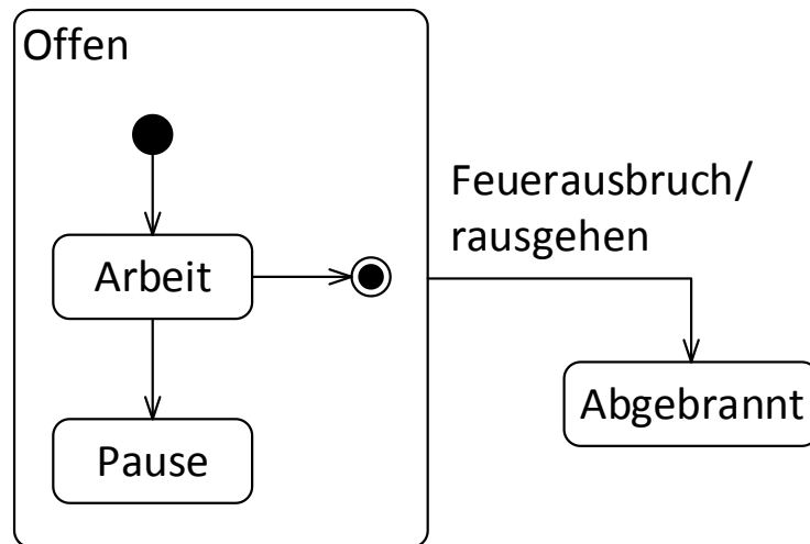
Abbildung 49: Verlassen eines zusammengesetzten Zustands mithilfe eines Events
