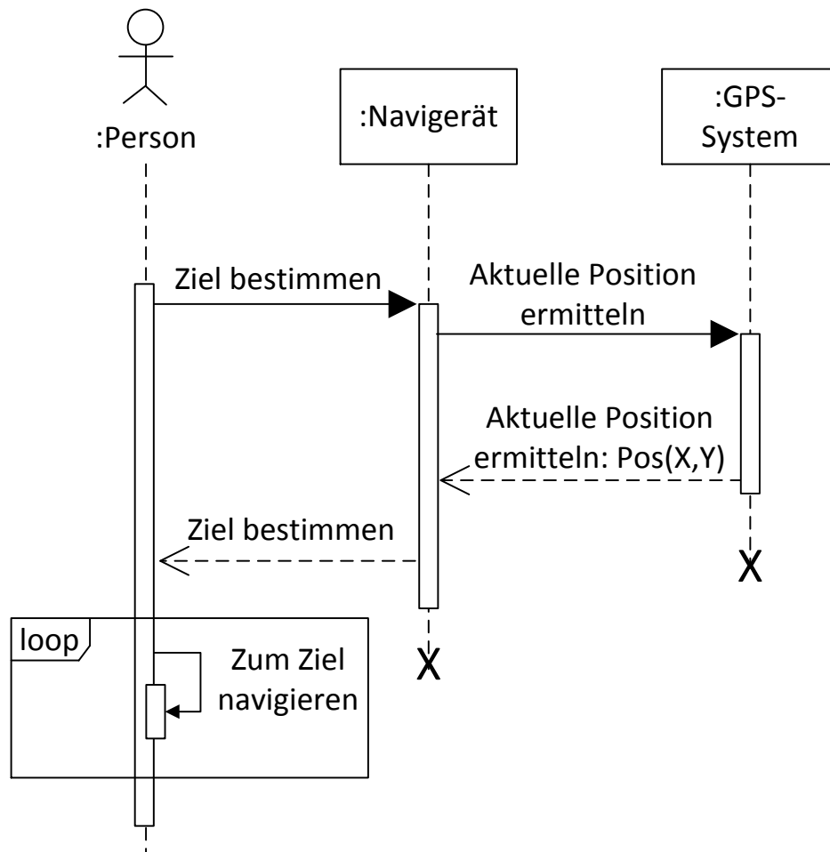
Abbildung 69: Sequenzdiagramm des Navigationsbeispiels
