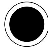
Abbildung 38: Endzustand
