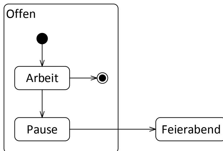
Abbildung 50: Direktes Verlassen eines zusammengesetzten Zustands
